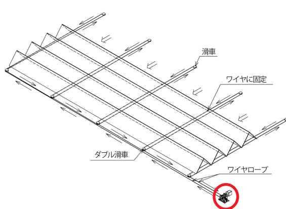
▲ 大型テント屋根開閉例
