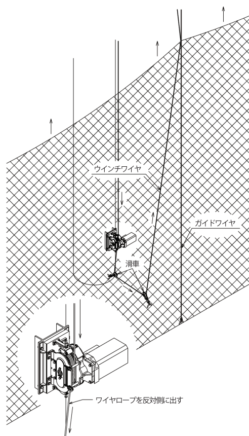
▲ ネット昇降例
