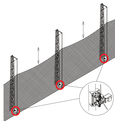
▲ ゴルフ練習場ネット昇降例
