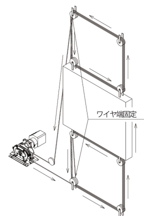
▲ ダンパー昇降例
