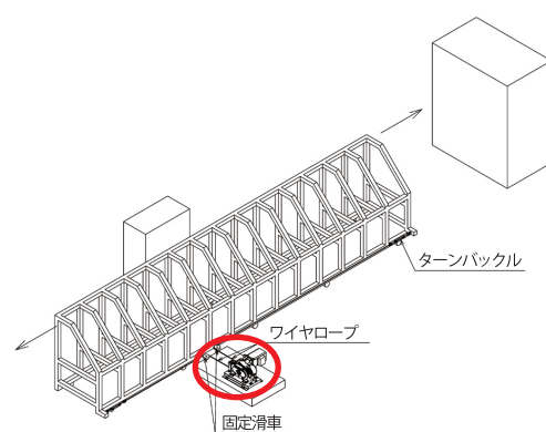
▲ 門開閉例
