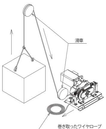
▲ 吊り下げ例
