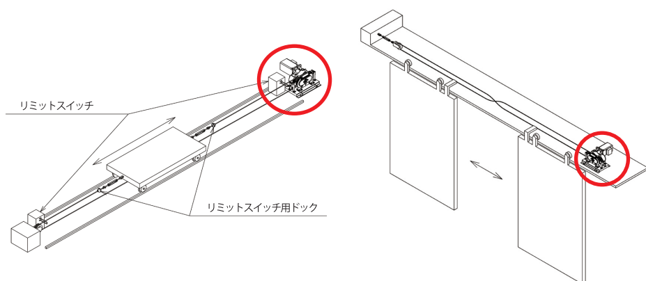
▲ 台車横行例
